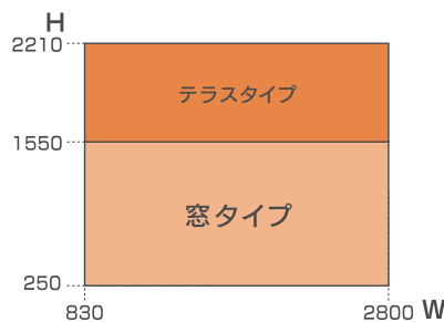
上げ下げ
