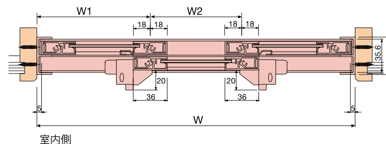
3枚建 Eタイプ
