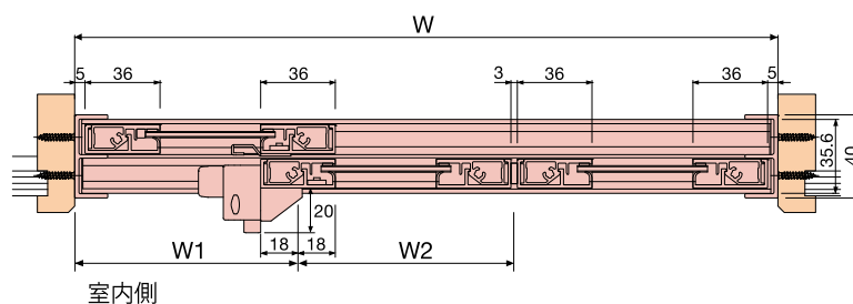
〔横断面納まり図〕
