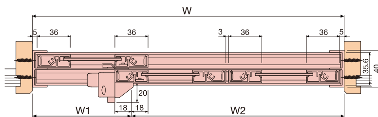
[ 横断面納まり図 ]
