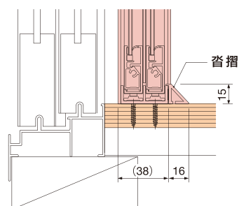
テラス沓摺納まり図 (オプション)
