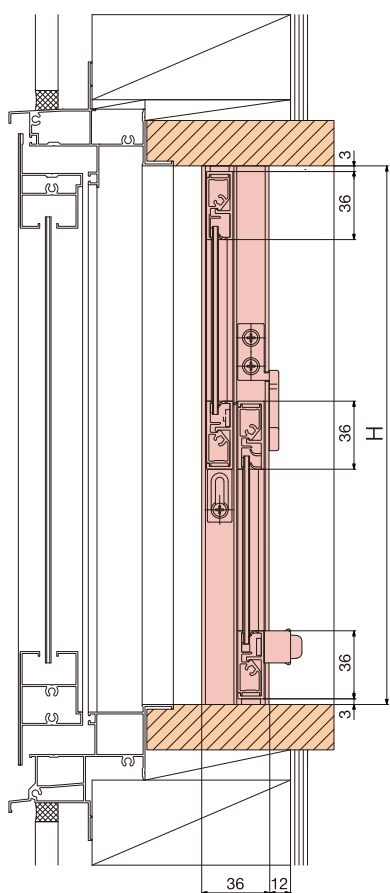
〔縦断面納まり図〕
